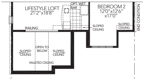
LOFT ELEV. A
